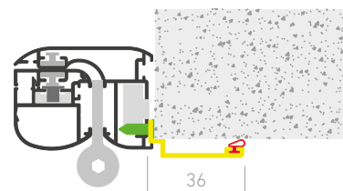
Puerta abatible Solape
